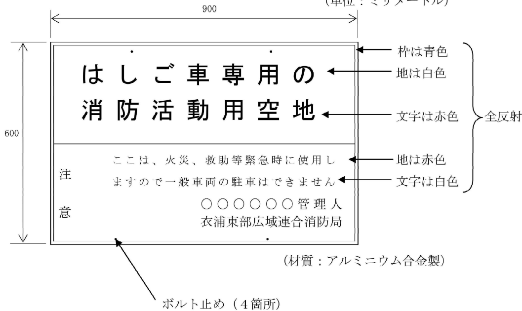
別図第2（第4条関係） 空地の規制標識
