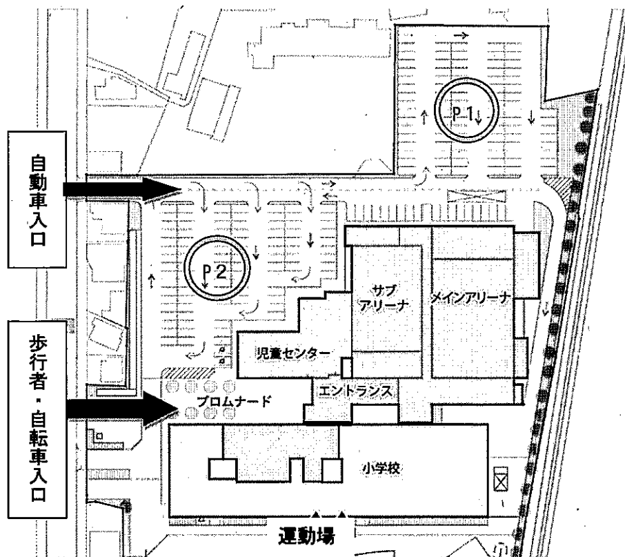
＜高浜小学校 平面図＞
