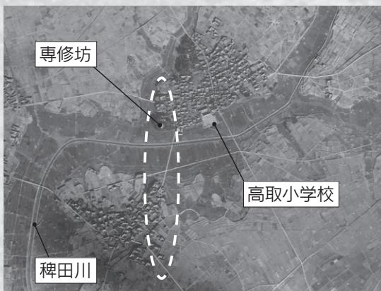
▲高取地区で三河地震の被害が大きかったとされる範囲(点線部分) ※国土地理院空中写真(昭和22年)に一部加筆
